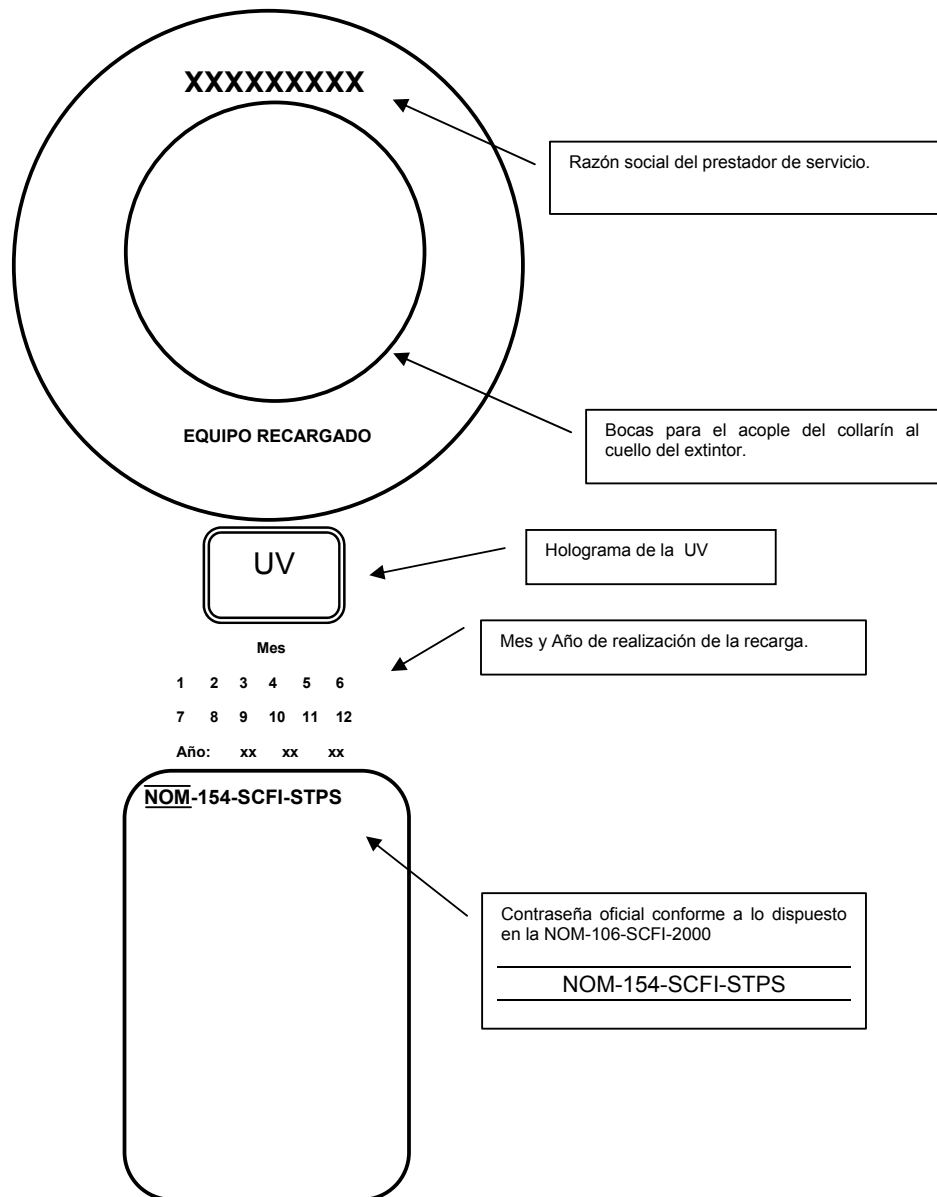
Figura 2.- Collarín
